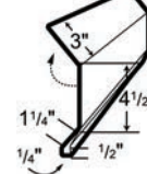
LG 130 SLIDING DOOR DRIP CAP
